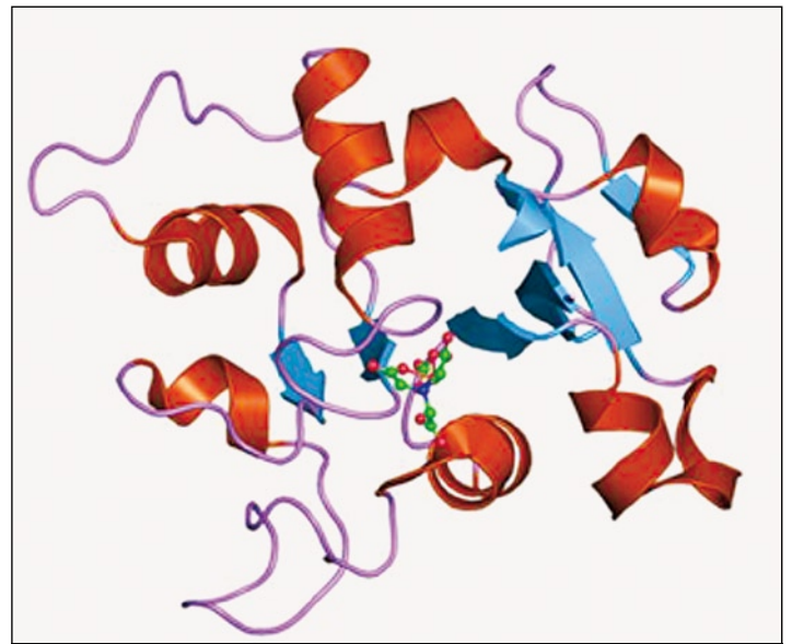
Obr. 3 – Molekula bielkoviny ovotransferrinu (conalbumin)
