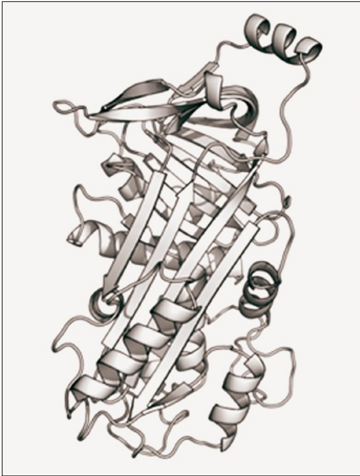
Obr. 2 – Molekula bielkoviny ovoalbuminu (ovalbumin)
